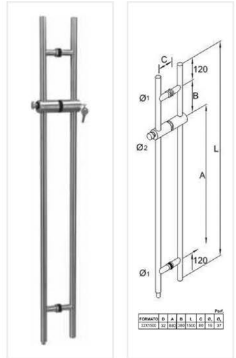
Jaladera con chapa de llave integrada. Acabado: Satín.
