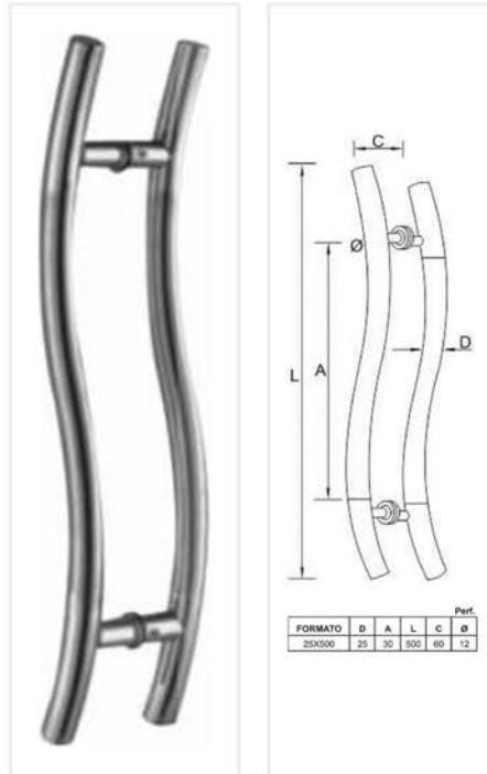
Jaladera tipo "S" Acabado: Satín y cromo.
