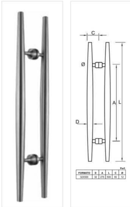
Jaladera tipo "H" con terminación punta de lápiz. Acabado: Satín.
