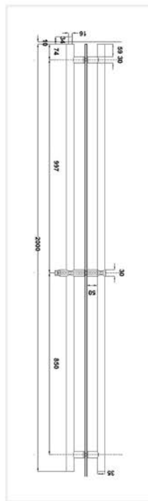
Jaladera tipo H con chapa al centro y seguro.
