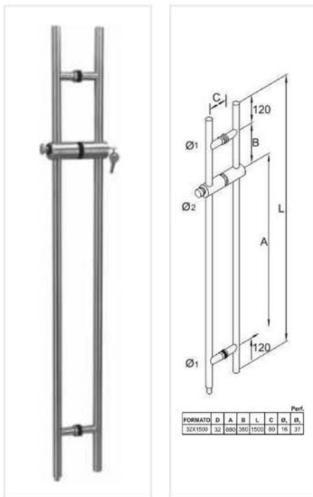
Jaladera con chapa de llave integrada. Acabado: Satín.
